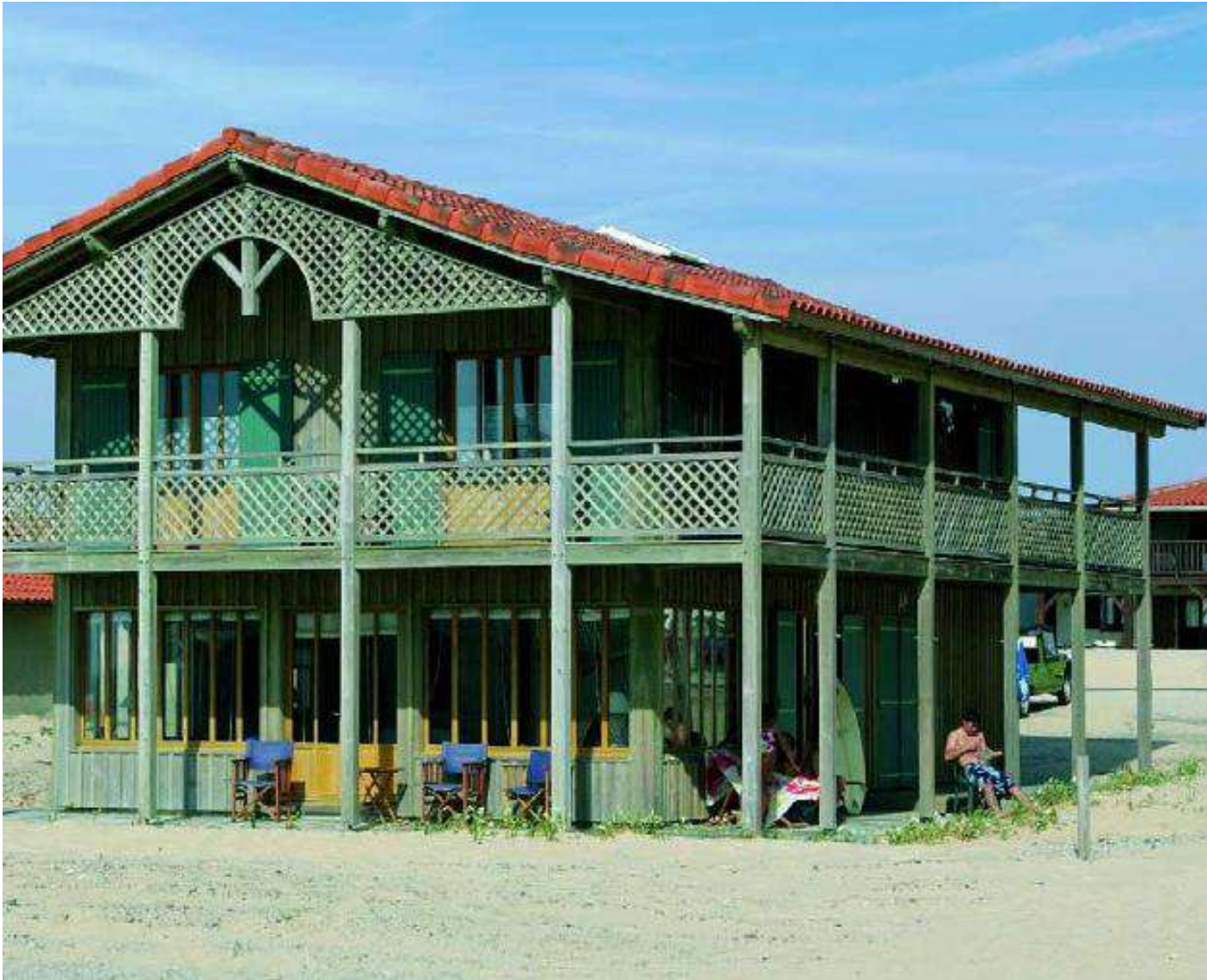
Madera aserrada estructural de pino pinaster. Saint Giron, France.
